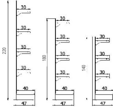
Duvar Üniteler Wall Unit
