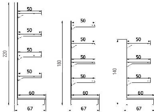
Duvar Üniteler Wall Unit
