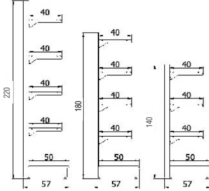
Duvar Üniteler Wall Unit
